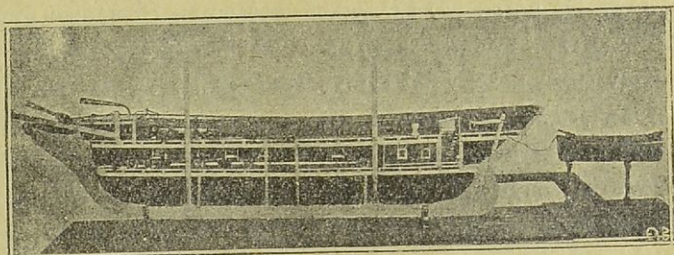
Τομὴ πυρπολικῆ (κατὰ τὸν κ. Ράδον).
