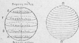
Σχ. 19. Παράλληλοι.
