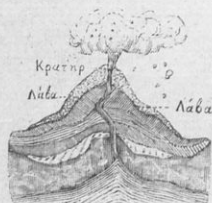
Σχ. 33. Ήφαιστειον.
