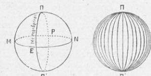
Σχ. 20-21 Μεσημβρινοί.
