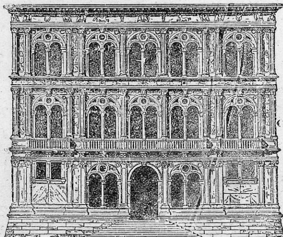
Palazzo Vendramin Calergi (Βενετία), μέγαρον ἀναγεννήσεως τοῦ οικοδόμου ἐτέλους 15 ου αἰῶνος. Ἐὐθυγραμμία, κανονικά τόξα ἐνθυμίζουν τὴν ρωμαϊκὴν τεχνοτροπίαν, κίονες κορινθιακοί.
