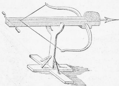
Σχορπιὸς (ἀναπαράστασις) ρίπτει βέλη
