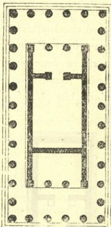
Εἰκ. 39. Ναὸς ἀμφιπρόστυλος. Εἰκ. 40. Ναὸς περίπτερος.
