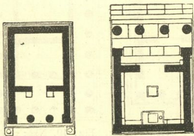
Εἰκ. 37. Ναὸς ἐν παραστάσι. Εἰκ. 38. Ναὸς πρόστυλος.
