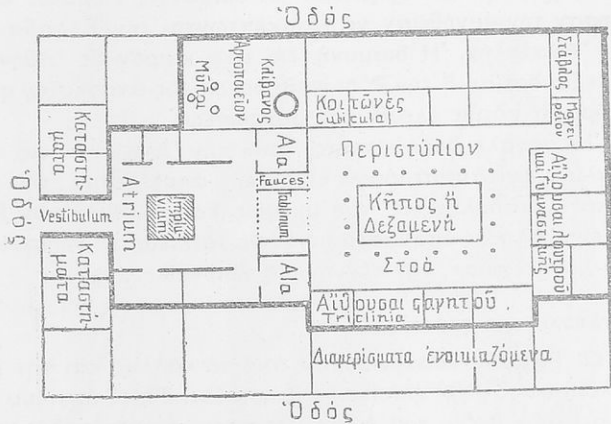
Σχέδιον ἑλληνορωμαϊκῆς οἰκίας
