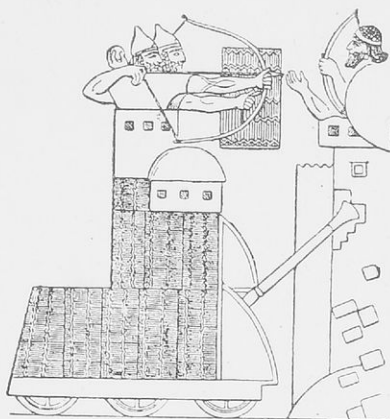
Πύργος ἐπὶ βάσεως τροχοφόρου (Πολιορκία τείχους)
