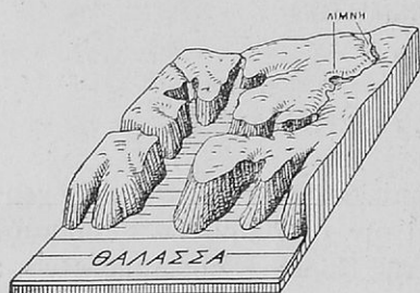
Διάγραμμα ἐμφαίνον τὴν ἀνάγλυ- φον μορφὴν ἑνὸς φιόρδ.
