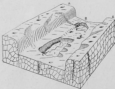
Ἡ μορφή τοῦ Κάρστ τῆς Γιουγκοσλαβίας. (1 πολιέ, 2 ντολίναι, 3 πηγαί, 4 καταβόθραι).
