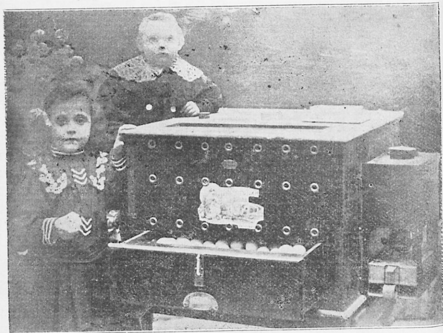
Εἰκ. 32. Κλωσσομηχανὴ διὰ θερμοῦ ὕδατος.
