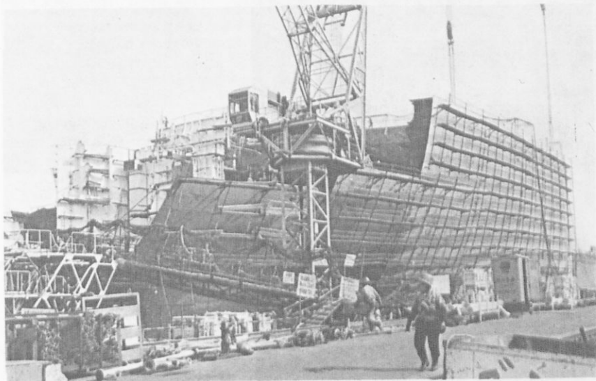
Ἡ ναυπήγηση ενός γιγάντιου καραβιού.
