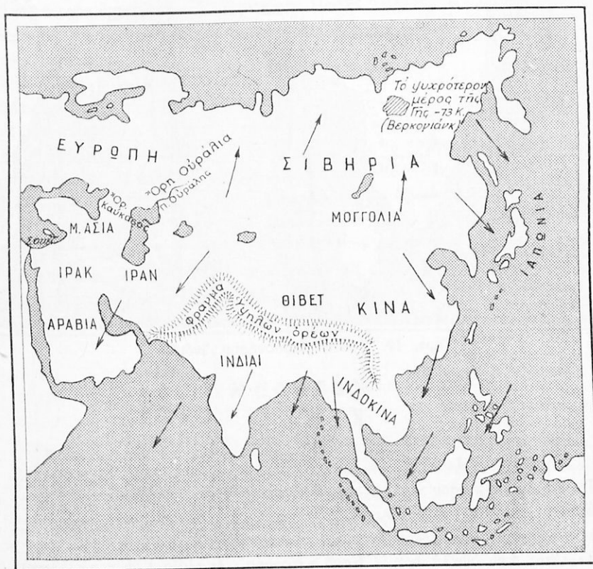
Χαρτ. 18. Χειμερινοὶ μουςσῶνες.
