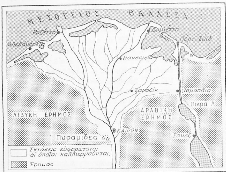
Χαρτ. 36. Τὸ Δέλτα τοῦ Νείλου.
