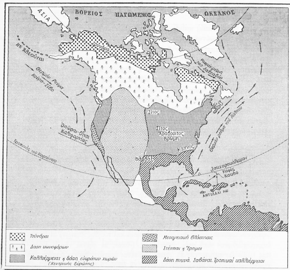
Χαρτ. 53. Βλάστησις εἰς Βόρειον καὶ Κεντρικὴν Ἀμερικὴν.
