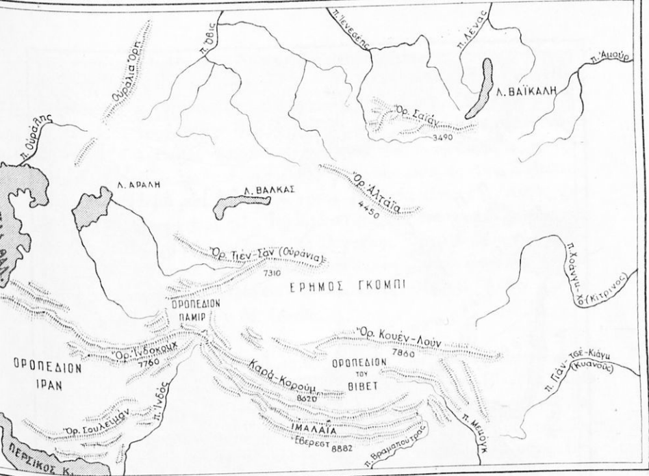
Χαρτ. 28. Αί υψηλότεραι όροσειραι καί ύψηλότερα όροπέδια 'Ασίας.
