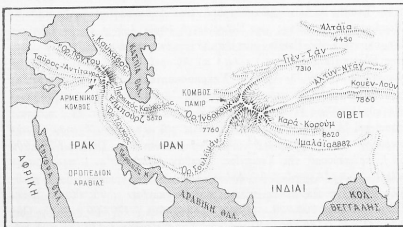
Χαρτ. 26. Ὁροσειραὶ τῆς Ἀσίας.
