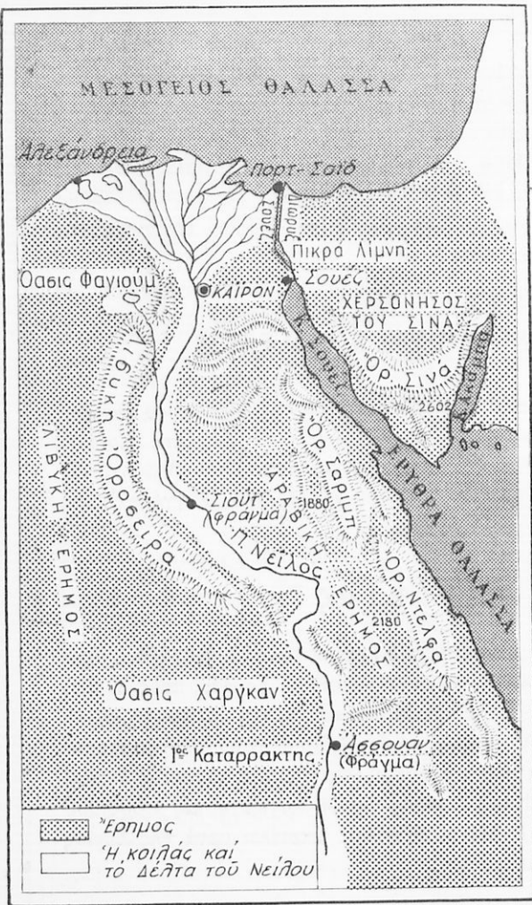
Χαρτ. 34. Αίγυπτος: Φυσικά περιοχαί.
