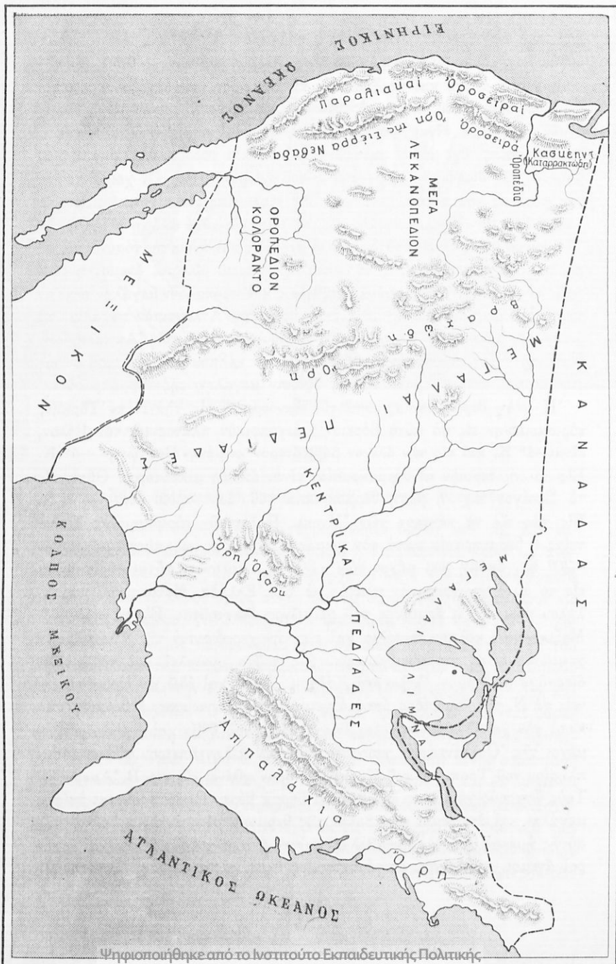
Χάρτ. 56. Πεδιάδες 'Ην. Πολιτειών 'Αμερικής.
