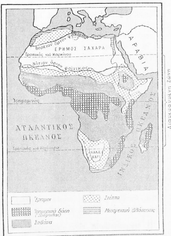
Χαρτ. 52. Διακεκαυμένη Ζώνη.
