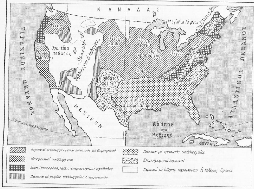
Χαρτ. 58. Γεωργικαὶ καὶ κτηνοτροφικαὶ περιοχαὶ Ἡν. Πολιτειῶν Ἀμερικῆς.
