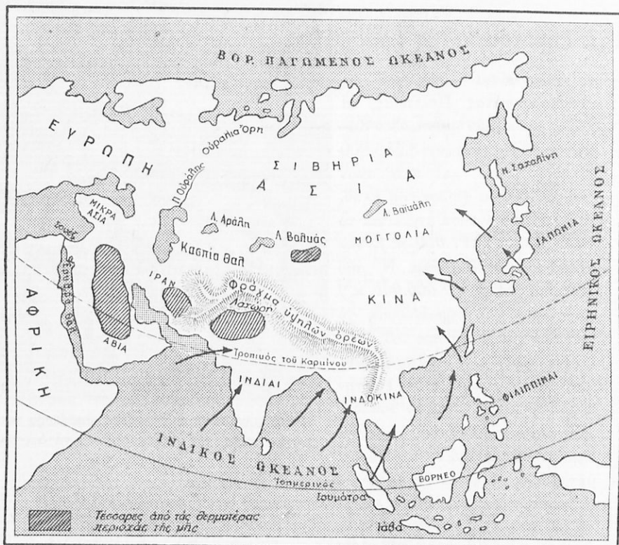
Χαρτ. 17. Θερνοί μουσδῶνες.
