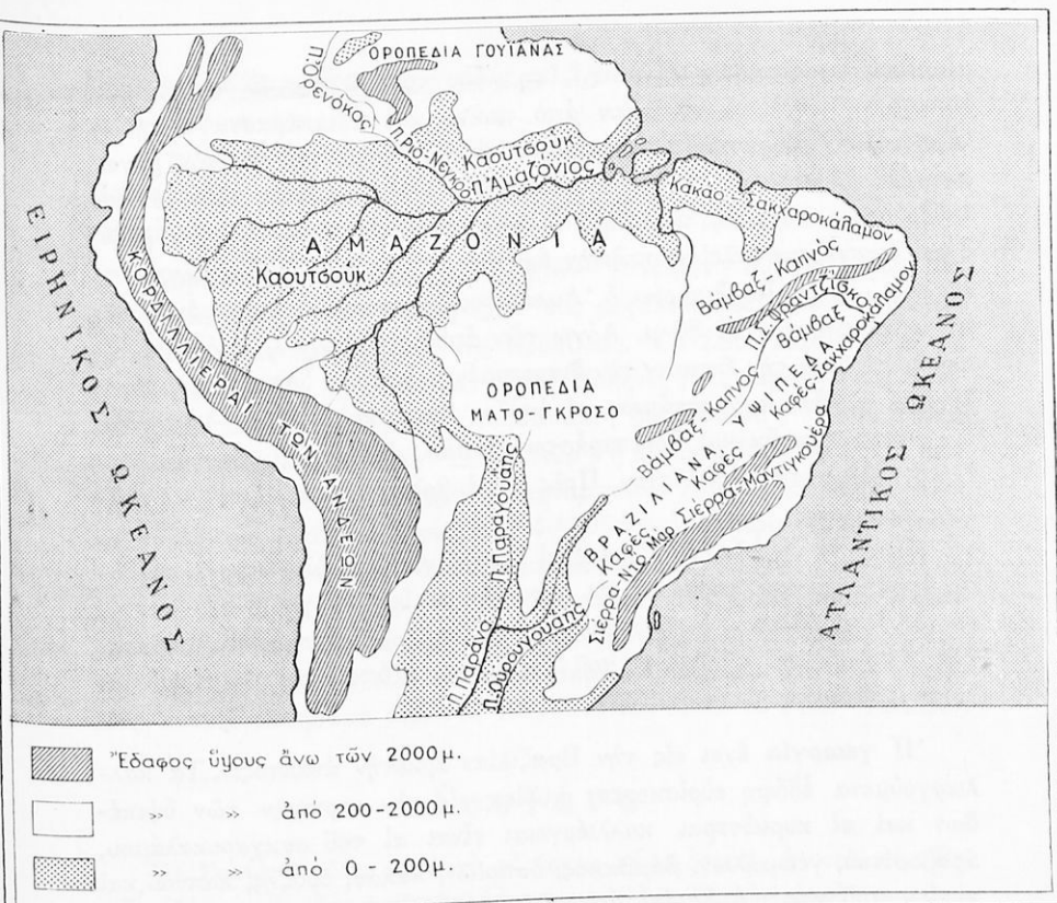
Χαρτ. 67. Μορφολογία εδάφους Βραζιλίας.
