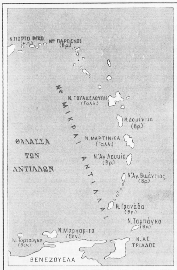
Χαρτ. 64. Μικραὶ Ἀντίλλαι.
