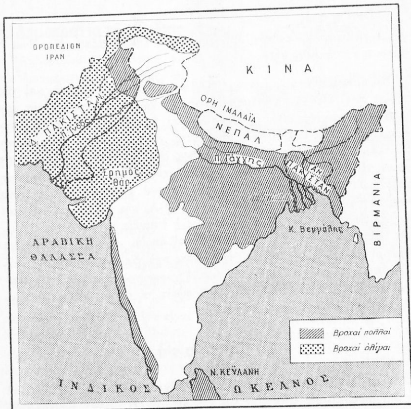
Χαρτ. 16. Κατανομή βροχῶν εἰς Ἰνδίας.
