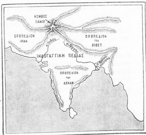
Χαρτ. 27. Ἡ διαμόρφωσις τοῦ ἐδάφους τῶν Ἰνδιῶν.
