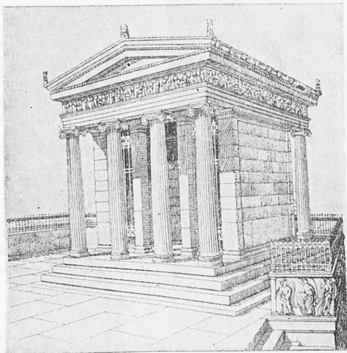
Ὁ ναὸς τῆς Ἀθηνᾶς ( Ἀπτέρου ) Νίκης, ἰωνικοῦ ρυθμοῦ ( Ἀναπαράστασις )
