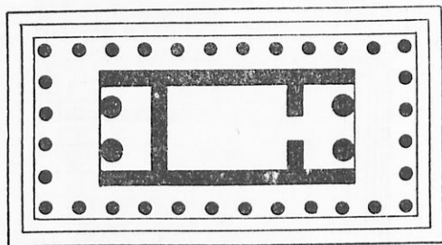
Σχ. 4. Ναὸς περίτερος
