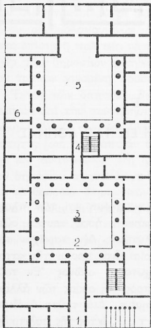
Σχέδιον ἀρχαίας οἰκίας
