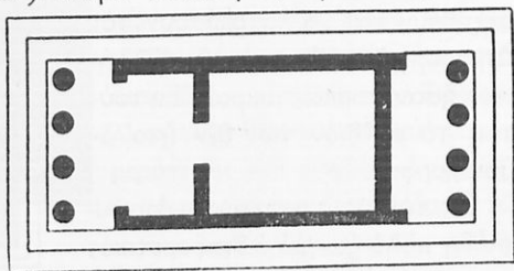
Σχ. 3. Ναὸς ἀμφιπρόστυλος
