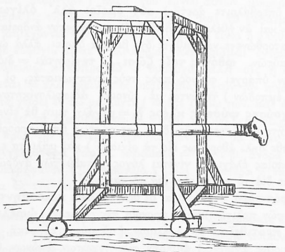
1. Κριός κρεμαστός.
