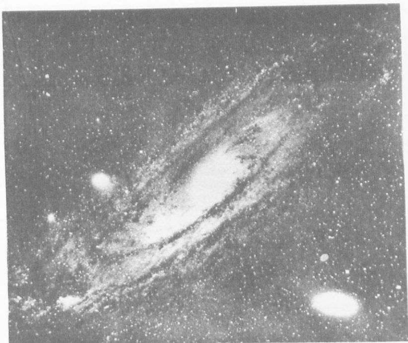
‘Ο νεφελοειδής της ‘Ανδρομέδας.
