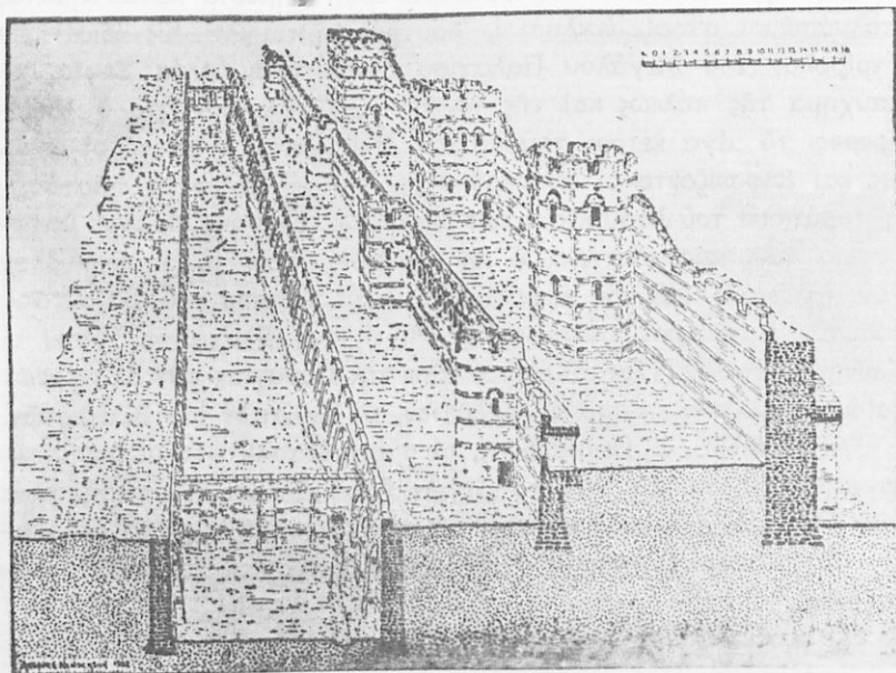
Σχεδιάσμα τῶν Θεοδοσιανῶν τειχῶν τῆς Κωνσταντινουπόλεως.
