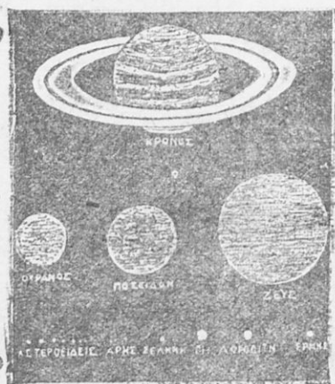
Σχ. 6. Σύγκρισις τοῦ μεγέθους τῶν πλανητῶν.
