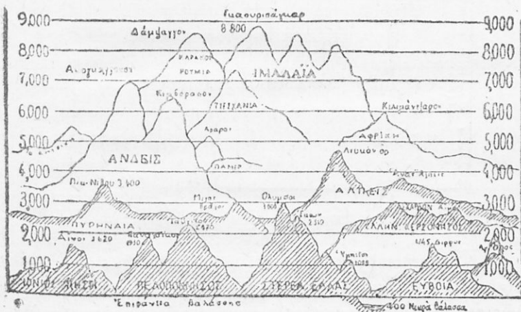
Σχ. 11. Ὅροσειραὶ καὶ κορυφαὶ διαφόρων ὑψών.
