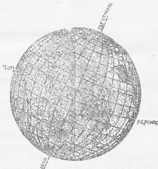
Σχ. 5. Κλίσις τῆς γῆς. — Φωτισμός αὐτῆς ὑπὸ τοῦ ἡλίου κατὰ τὴν θερμὴν τροπὴν.
