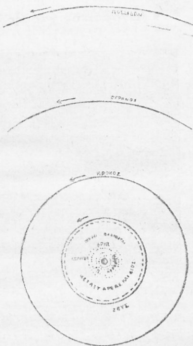
Σχ. 7. Τὸ ἡλιακὸν σύστημα.
