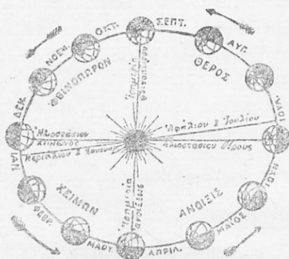
Σχ. 4. Ἡ περιφορὰ τῆς γῆς περὶ τὸν ἥλιον.
