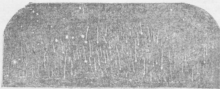
Σχ. 9. Βροχὴ διατιόντων ἀστέρων.
