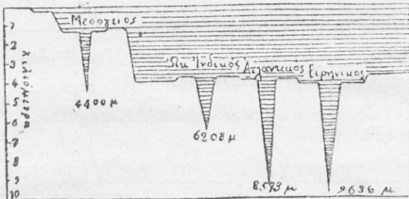
Σχ. 12. Τὰ βάθη τῆς θαλάσσης.
