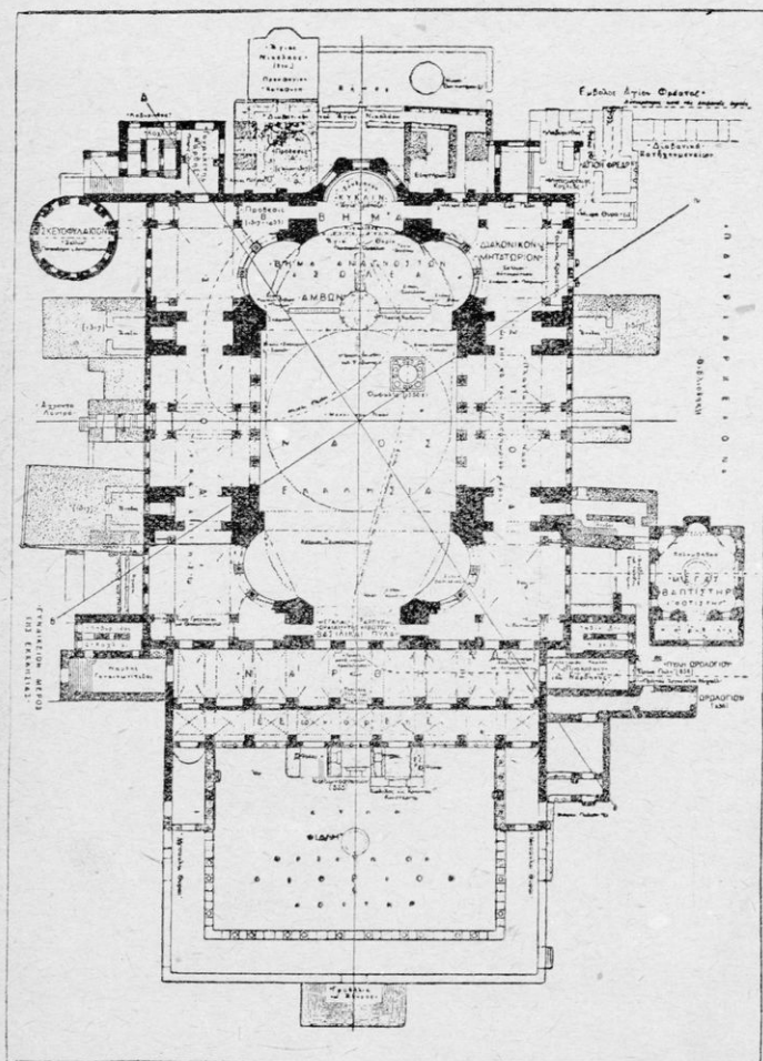
Εἰκ. 16. Κάτοπις τοῦ Ναοῦ τῆς Ἁγίας Σοφίας.
