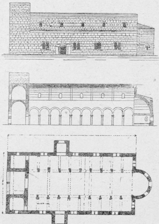
Εἰκ. 11. Δρομικὸς Ναός.
