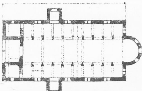
Εἰκ. 27. Δρομικός ναός.
