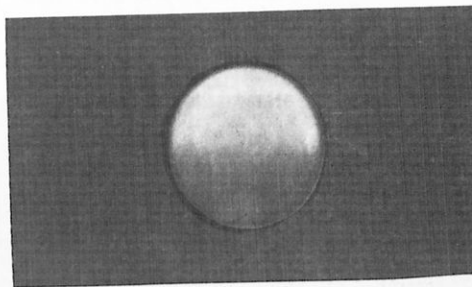
Ἡ Γῆ ὅπως φαίνεται ἀπὸ τή Σελήνη
