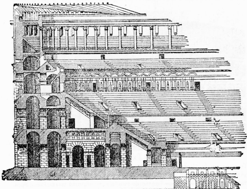
Τὸ Κολοσσαῖον. (Κάθετος τομὴ)
