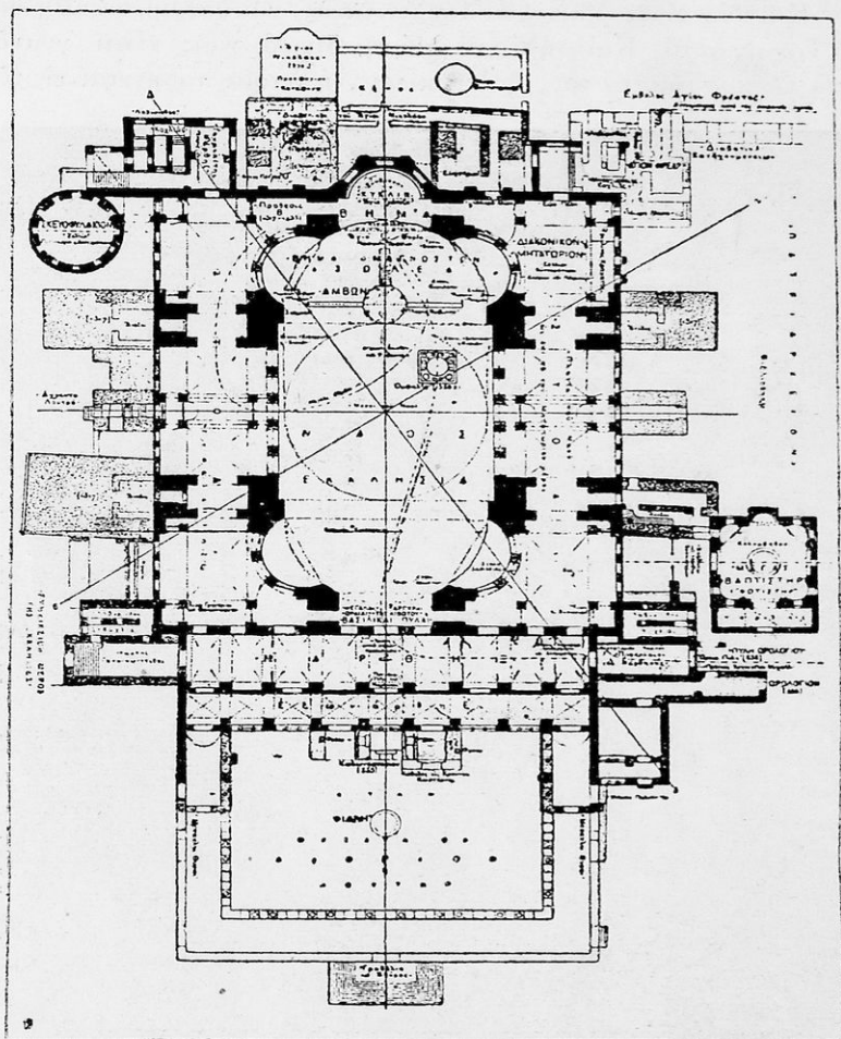
Εἰς. 32. Κάτοψις τῆς Ἀγίας Σοφίας.
