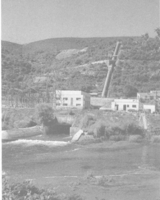
Ὑδροηλεκτρικό ἐργοστάσιο Ἄγρα
