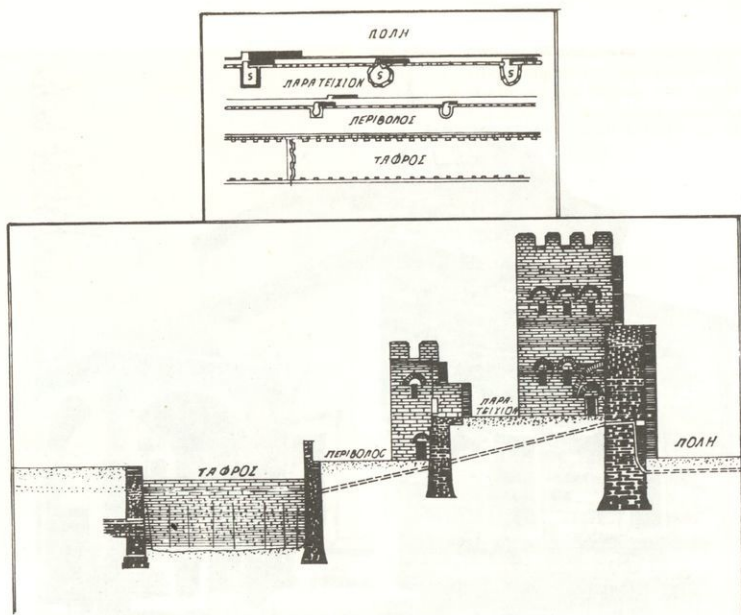
Τὸ τεῖχος τοῦ Θεοδοσίου
