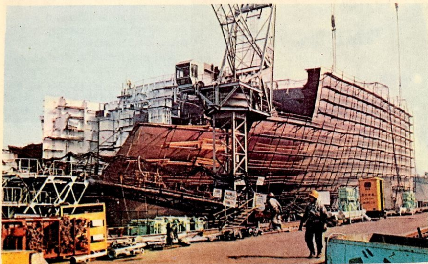
Ή ναυπήγηση ενός γιγάντιου καραβιού.
