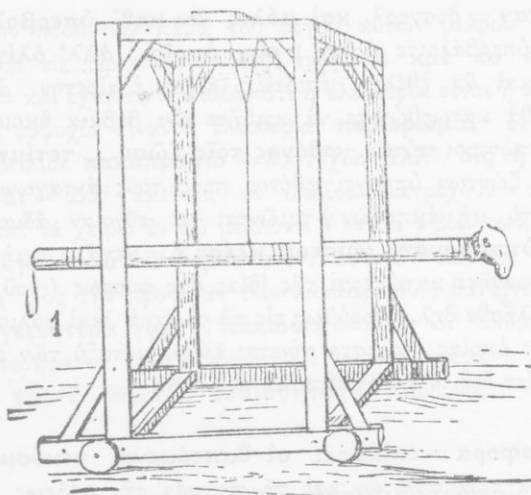
1. Κριός κρεμαστός.
