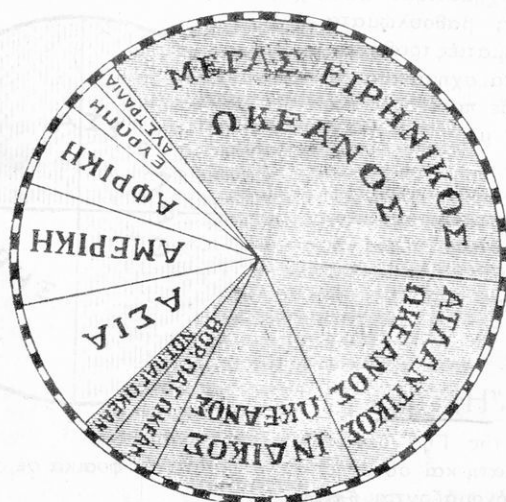
Είκ. 2. 'Ωκεανοί και ήπειροι
