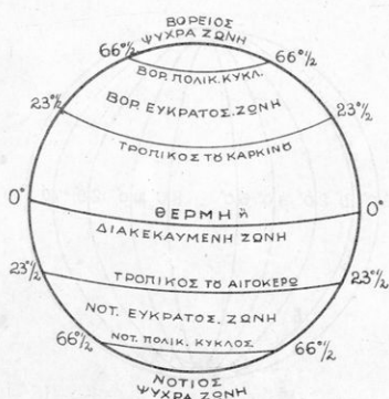
Εἰκ. 7. Ζώνες τῆς Γῆς
