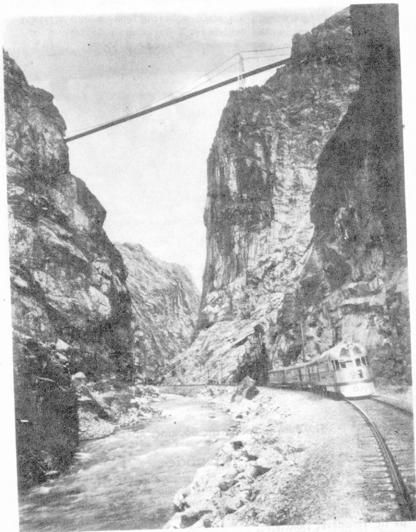
Εικ. 34 Γραφικόν τοπίον τοῦ Κολοράντο
