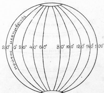
Εἰκ. 6. Μεσημβρινοὶ κύκλοι
