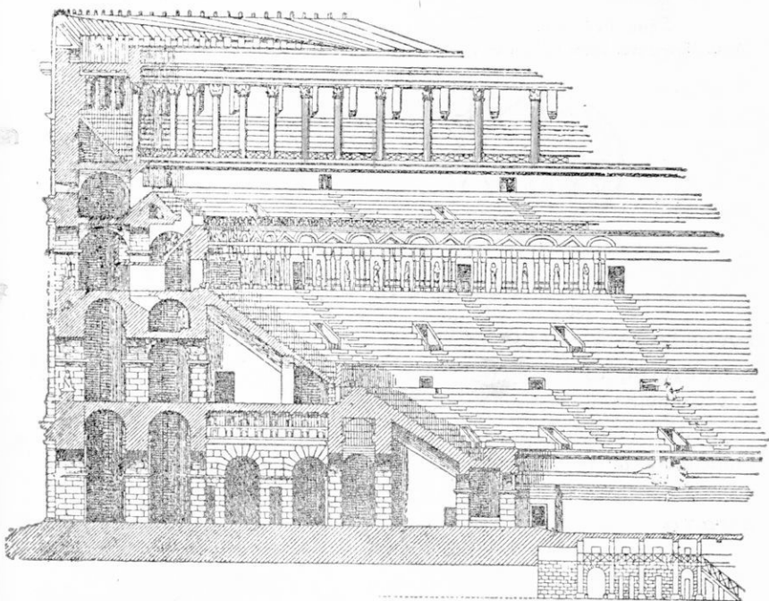
Τὸ Κολοσσαῖον (κάθετος τομή).
