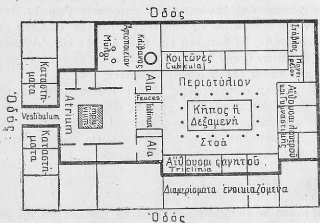
Σχέδιον ἑλληνορρωμαϊκῆς οἰκίας
