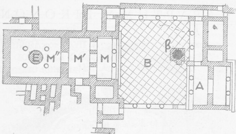
Εικ. 3. Σχέδιον μεγάρου.
