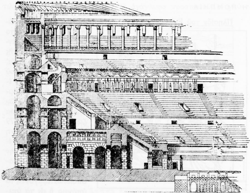
Τὸ Κολοσσαῖον. (Κάθετος τομὴ)
