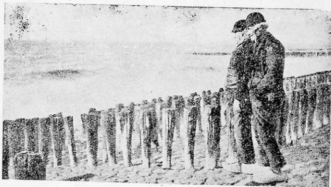
40. 'Ολλανδοί μέ τά ξύλινα παπούτσια τους μπροστά στά άτελείω- τα από ξύλινους πασσάλους φράγματα, πού έχουν φτιάσει για νά προστατεύσουν τόν τόπο τους από τίς θαλάσσιες πλημμύρες.
