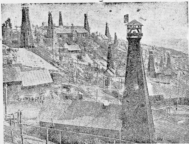
23. Πετρελαιοπηγές στη Ρουμανία. Οί ξύλινοι πύργοι κρύβουν την άντλία που άνεβάζει το πετρέλαιο από τα βάθη της γης.
