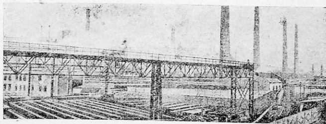
54. Τὸ Ντόρτμουντ , βιομηχανικὴ πόλη τῆς Γερμανίας.
