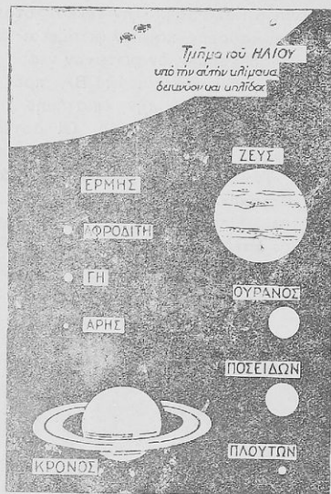
Σχ. 14. Συγκριτικὸν μέγεθος τῶν πλανητῶν.
