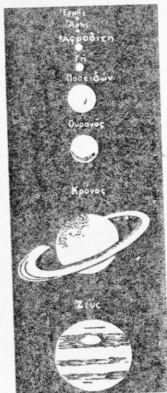
Εἰκ. 9. Ἡ Γῆ καὶ οἱ ἄλλοι πλανῆτες.
