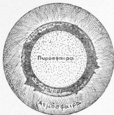
Εικ. 2. Λιθόσφαιρα και πυρόσφαιρα
