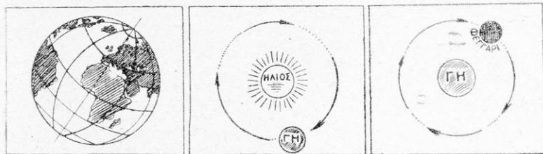
Εικ. 5. Περιφορά τῆς γῆς γύρω ἀπὸ τὸν ἥλιο.
