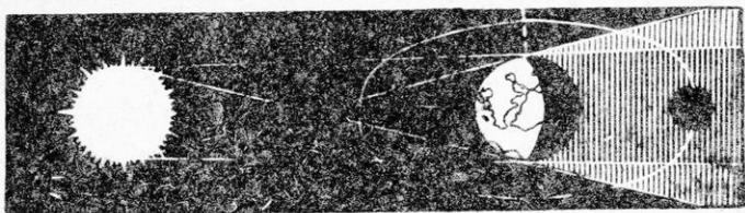
Εἰκ. 14. Ἐκλειψις Σελήνης
