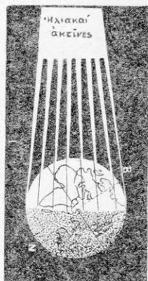
Εικ. 6. ‘Ημέρα και νύκτα.
