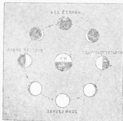
Εικ. 13. Φάσεις της Σελήνης
