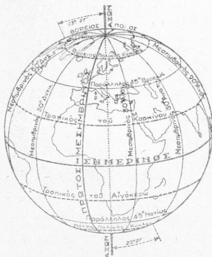
Εικ. 7. Ο άξονας της γης είναι κεκλιμένος
