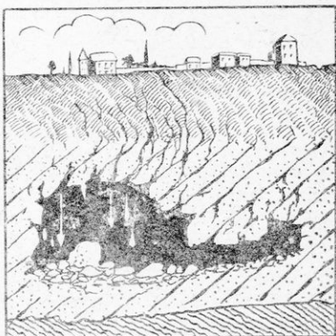
Εικ. 4. Τεκτονικοί σεισμοί
