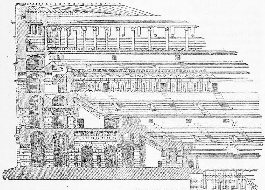
Τὸ Κολοσσαῖον (κάθετος τομή).
