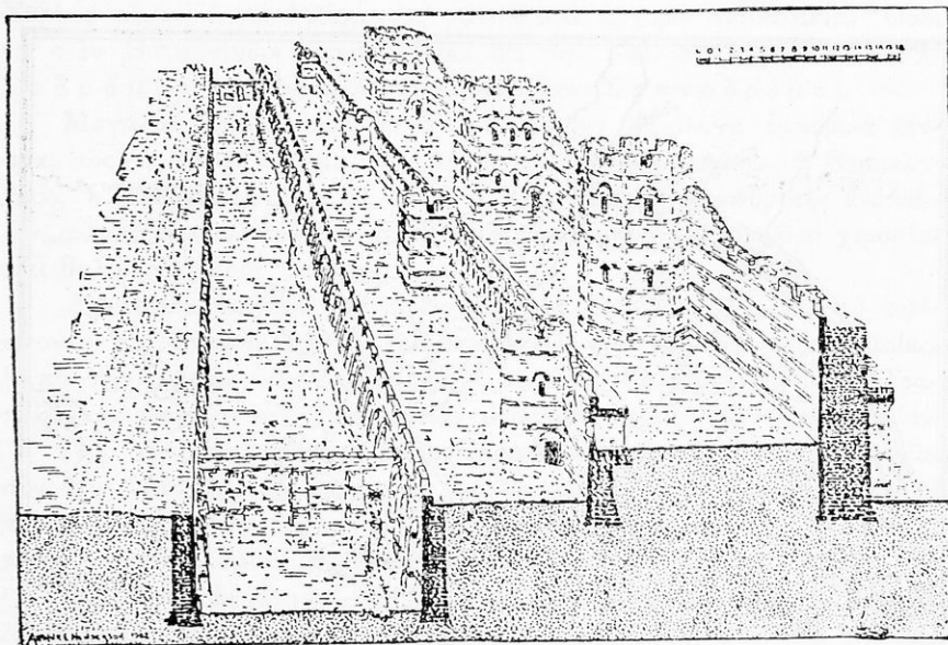
29. Τμῆμα τῶν τειχῶν τῆς Κωνσταντινουπόλεως
