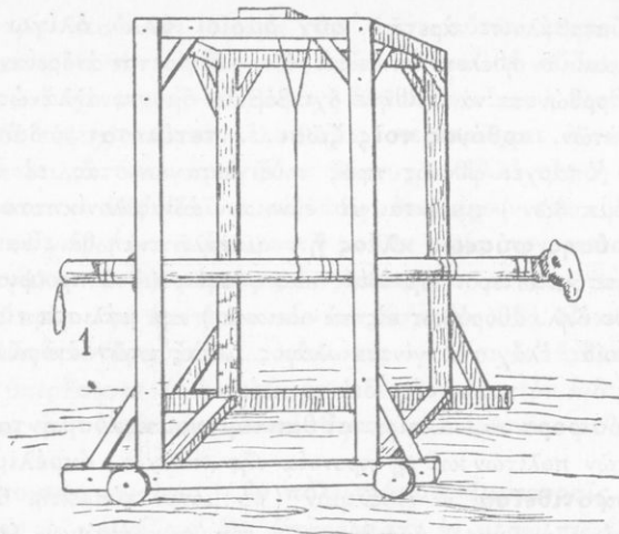
1. Κριός κρεμαστός.
