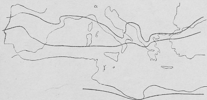
Εἰκ. 20. Χάρτης βροχῶν τῶν χωρῶν τῆς Μεσογείου.
