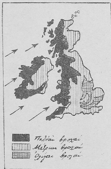
Εἰκ. 34. Χάρτης βροχῶν τῶν Βρεττανικῶν νήσων.
