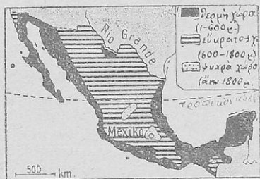
Εἰκ. 80. Κλιματολογικὸς χάρτης τοῦ Μεξικοῦ.
