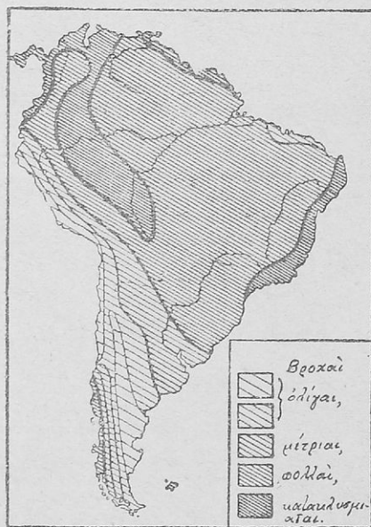
Εἰκ. 85. Χάρτης βροχῶν τῆς Νοτίου Ἀμερικῆς.
