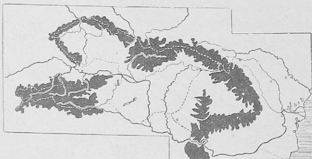
Εἰκ. 41. Αἱ χώραι τοῦ Δουνάβεως (Αὐστρία, Τσεχοσλοβακία, Οὐγγαρία, Ῥουμανία).
