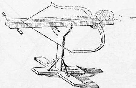
Σκορπιὸς (ἀναπαράστασις) ρίπτει βέλη.
