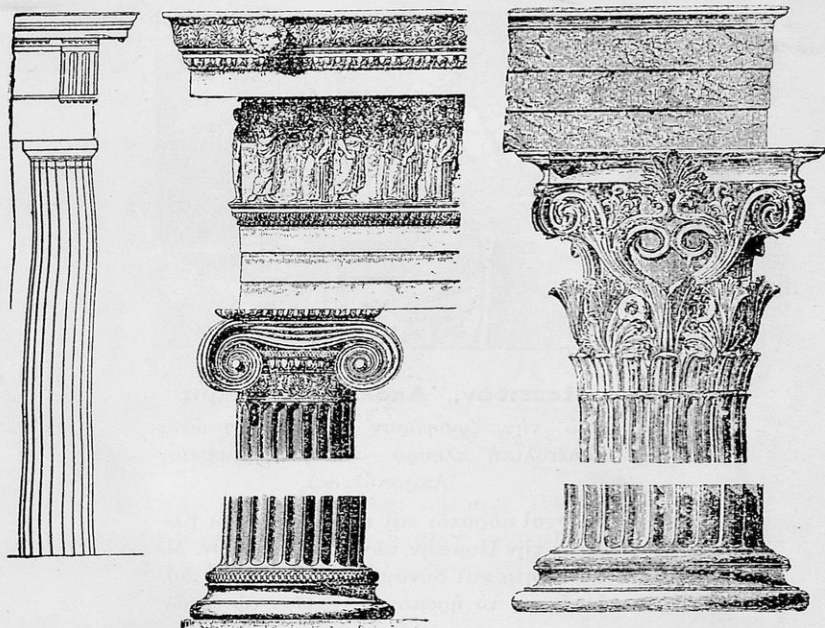
Κίονες, κατὰ σειράν δωρικός, ἰωνικός, κορινθιακός.
