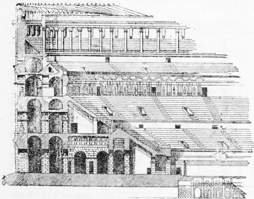
Τὸ Κολοσσαίου. (Καθετὸς τομῆ)
