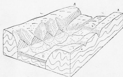
Γεωλογικὴ ἐξέλιξις ἐνὸς λεκανοπεδίου τῆς Βαλκανικῆς Χερσονήσου.
