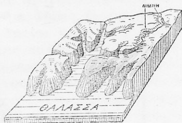
Διάγραμμα ἐμφαίνον τὴν ἀνάγλυφον μορφήν ἑνὸς φιορδ.
