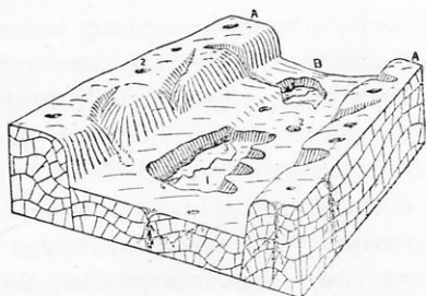
Ἡ μορφή τοῦ Κάροτ τῆς Γιουγκοσλαβίας. (1 πολιέ. 2 ντολίνα. 3 πηγαί. 4 καταβόθραι).
